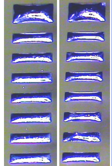
Links: Lötperlenbildung mit konventionellem VOC-freiem Flussmittel Rechts: 2009MLF
